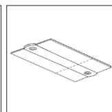
3FR.8010.xx XTSF 10 Afdekplaat
