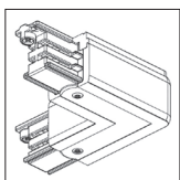
3FR.9340.xx XTS 34 Hoekstuk 90° vast
